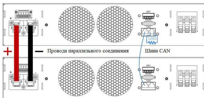
Рисунок 4 - Схема параллельного подключения двух приборов
