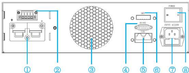
Рисунок 1 - Задняя панель
