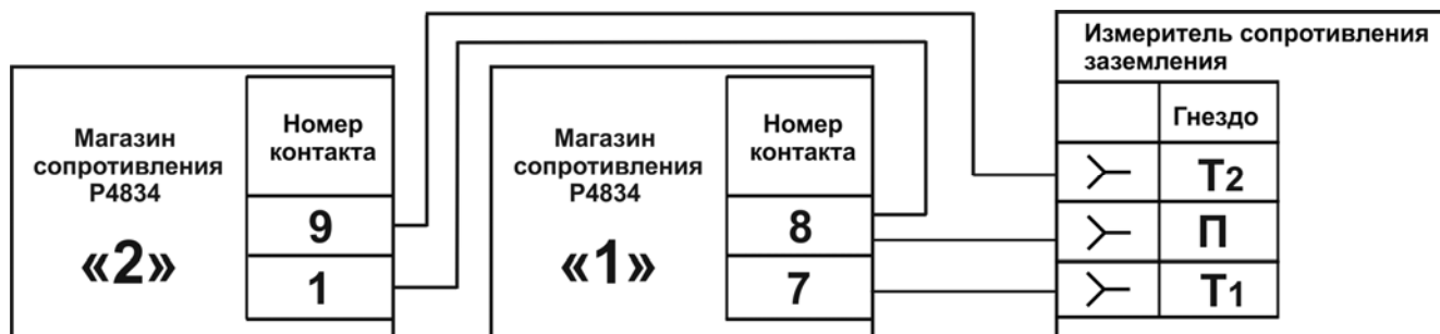
Рисунок 6.6.2 – Схема подключения при опробовании
