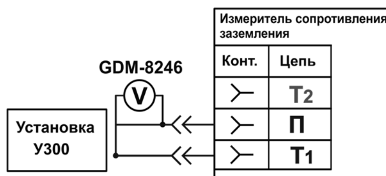
Рисунок 6.7.1 – Схемы определения погрешности измерений напряжения переменного тока
