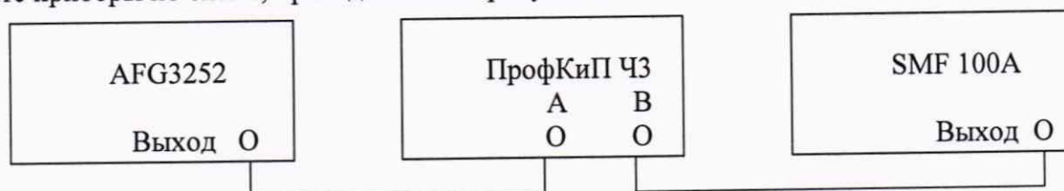
Рисунок 5 - Схема подключения приборов при определении диапазона измерения отношения частот
