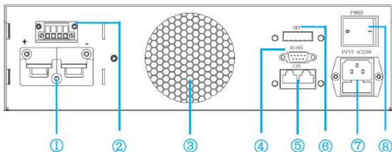
Рисунок 1 - Задняя панель
