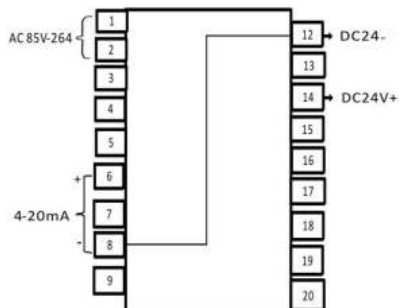
Рисунок 4 - Подключение к контроллеру (вариант 2)
