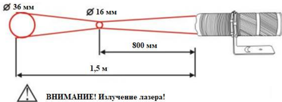
Рисунок 1 - Выбор оптимального расстояния для измерения
