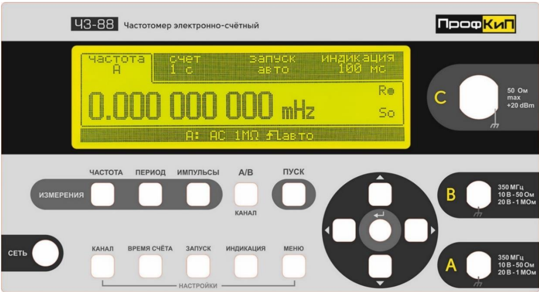
Рисунок 4. Внешний вид передней панели и расположение органов управления.
