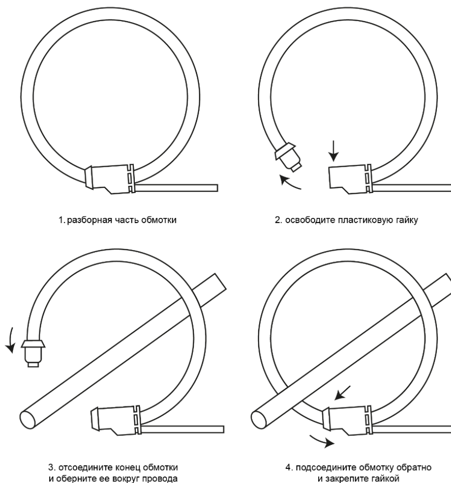
Рисунок 13 – Принцип установки Датчика вокруг провода
