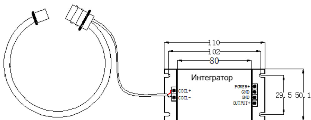
Рисунок 4 – Внешний вид датчика КСР-6 с 1 каналом подключения
