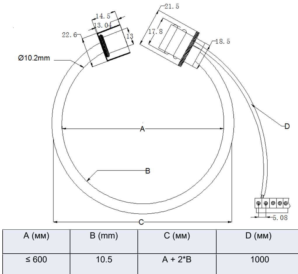
Рисунок 3 – Габаритные размеры гибкого измерительного кольца датчика КСР-6
