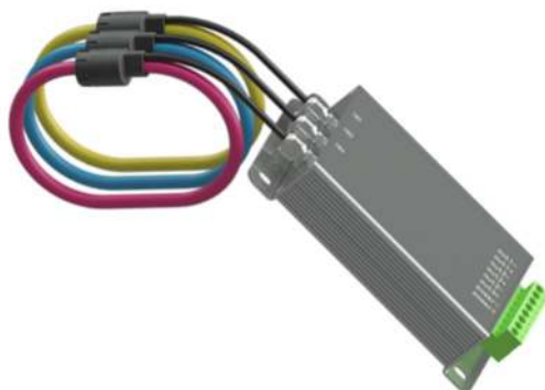
Рисунок 7 – Внешний вид датчика КСР-6 с 3 каналами подключения
