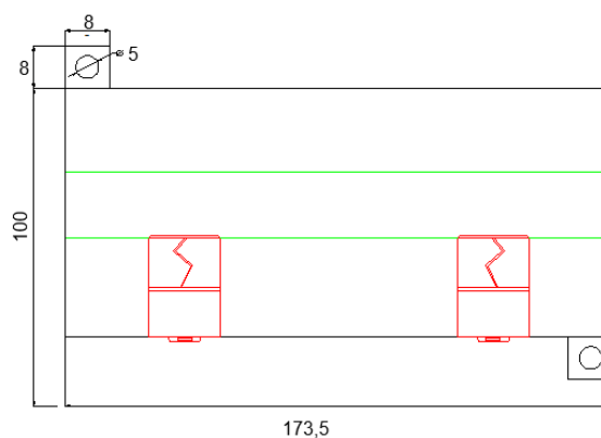
Рисунок 11 – Габаритные размеры интегратора для датчика КСР-6 с 12 каналами подключения
