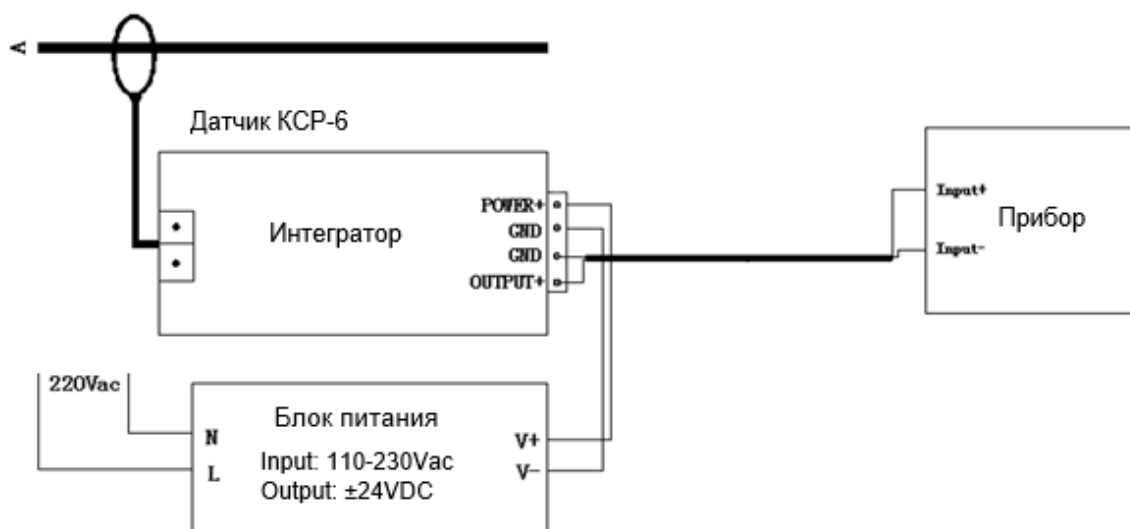
Рисунок 6 – Схема подключения для КСР-6 с 1 каналом подключения
