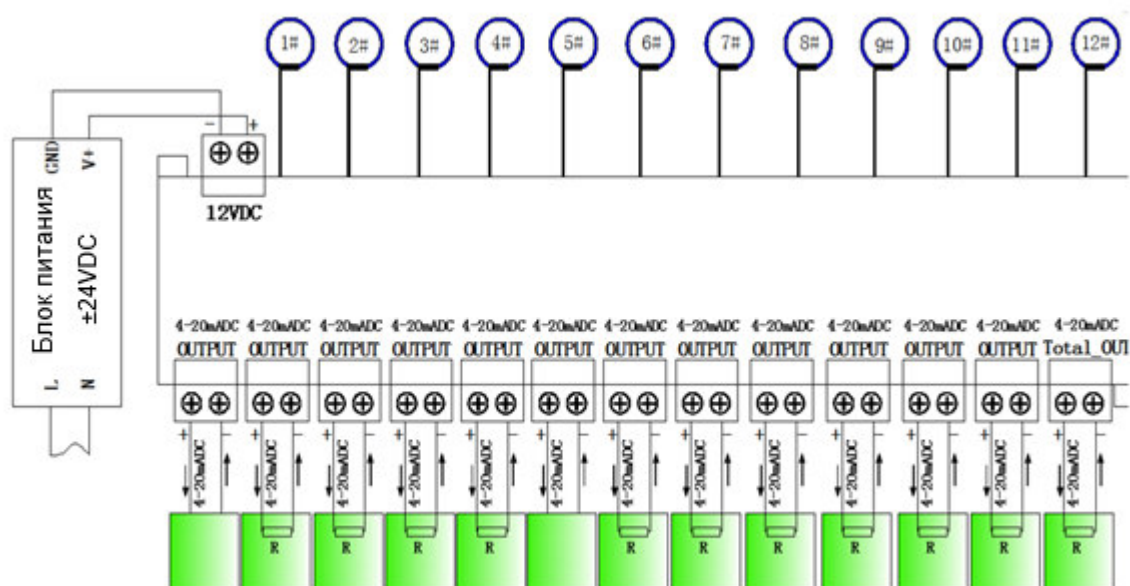
Рисунок 12 – Схема подключения для датчика КСР-6 с 12 каналами подключения
