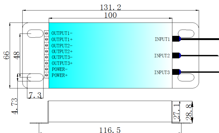
Рисунок 7 – Внешний вид датчика КСР-6 с 3 каналами подключения
