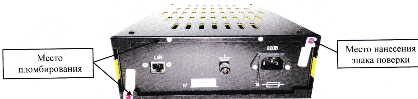
Рисунок 2 – Общий вид средства измерений, схема пломбирования от несанкционированного доступа, обозначение места нанесения знака поверки
