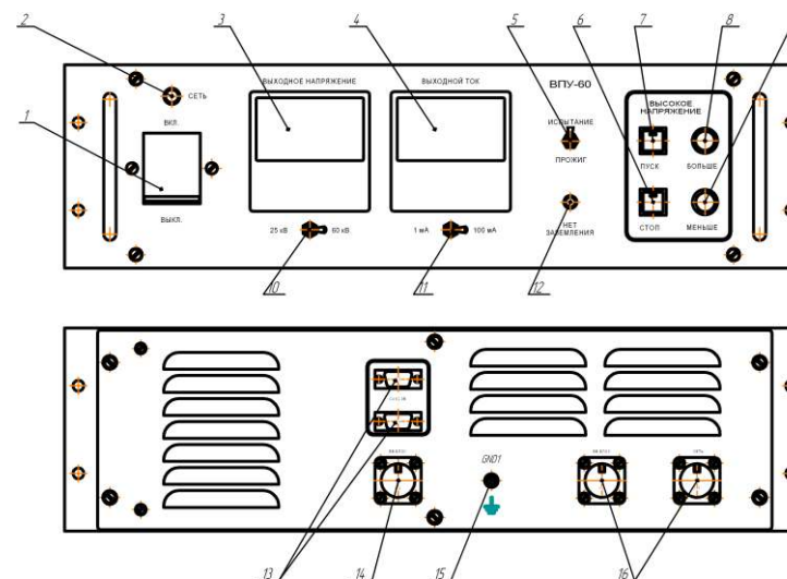
Рис. 2 Электронный блок
