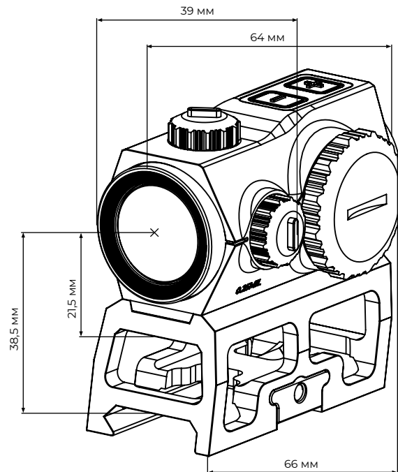
Размеры коллиматорного прицела RDC 1x20 с высоким кронштейном
