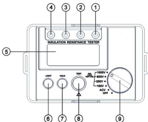
Рис.1 Передняя панель прибора
