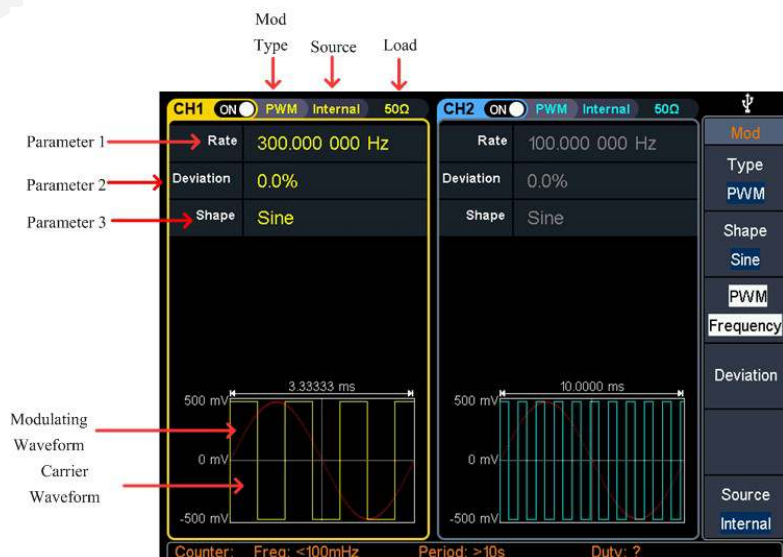
Рисунок 18 - Пользовательский интерфейс широтно-импульсной модуляции
