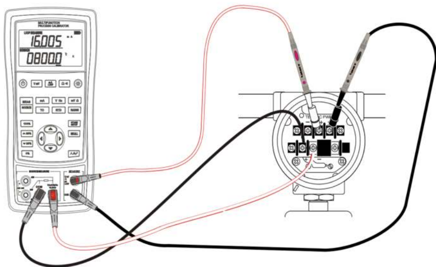
Рисунок 29 - Подключение калибратора
