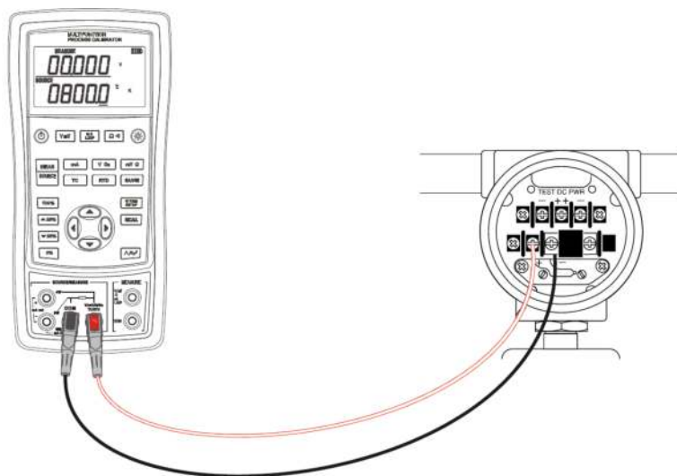
Рисунок 27 - Схема подключения
