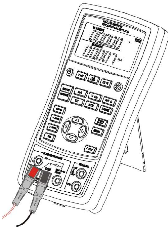
Рисунок 13 - Коммутация
