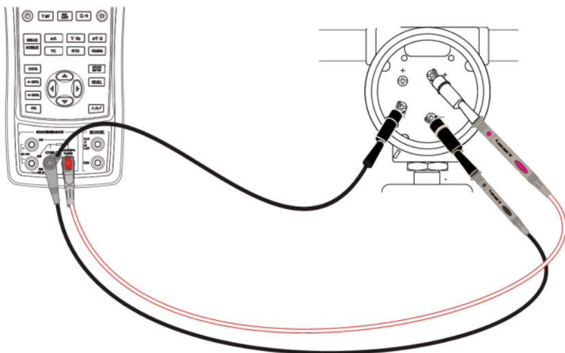
Рисунок 28 - Схема соединения
