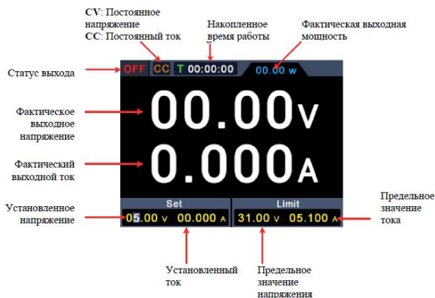
Рисунок 4 - Пользовательский интерфейс
