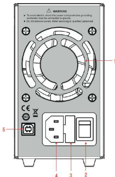
Рисунок 3 - Обзор задней панели
