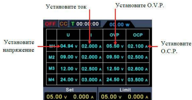
Рисунок 7 - Сохранение и вызов настроек сигнала
