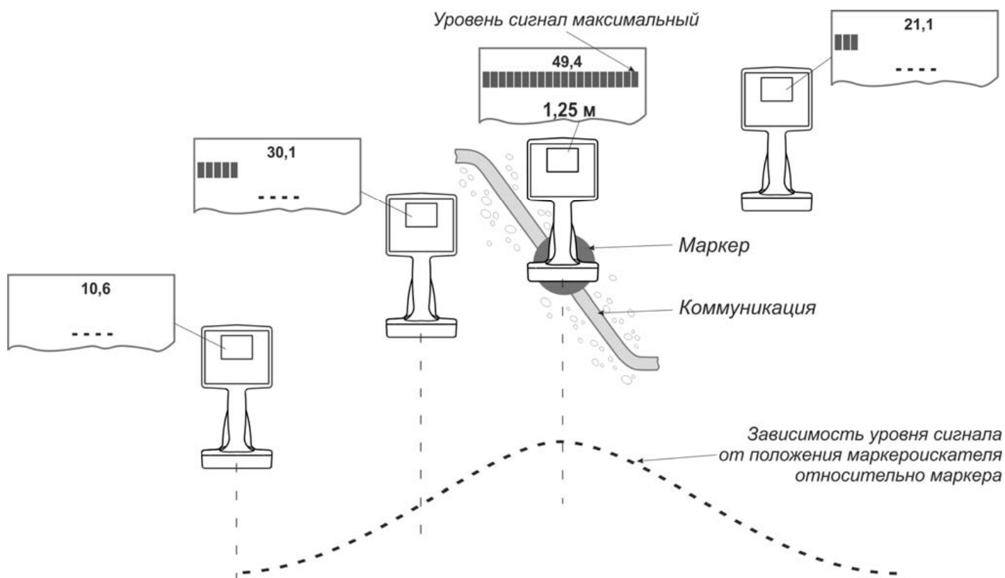
Рисунок 3.26 – Зависимость уровня сигнала от положения маркероискателя
