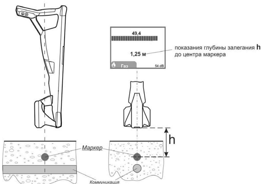
Рисунок 3.2 в – Определение глубины залегания
